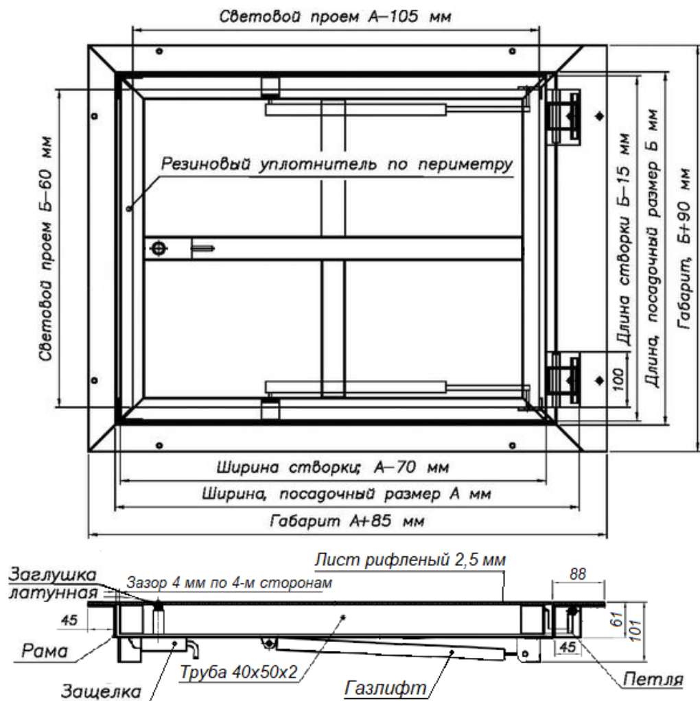
Рисунок 1 - Параметры напольного люка ЛНСП.
