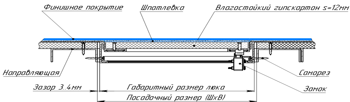
Схема монтажа люка ЛПНШ
