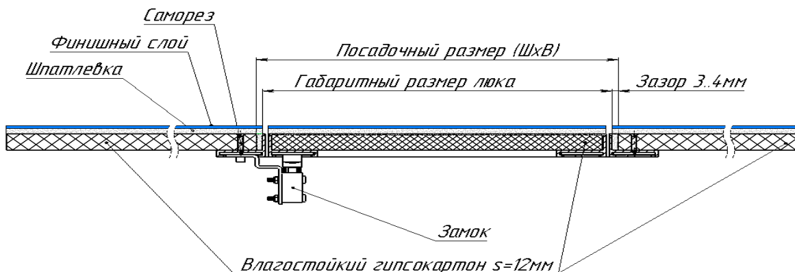
Схема монтажа люка ЛПНШ
